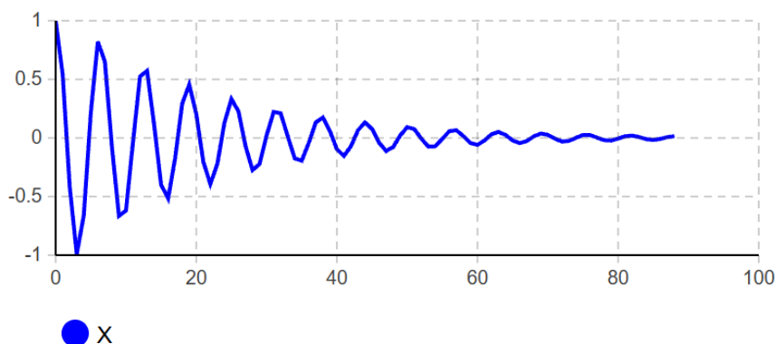
Рисунок 2 – График зависимости смещения грузика x от времени.
